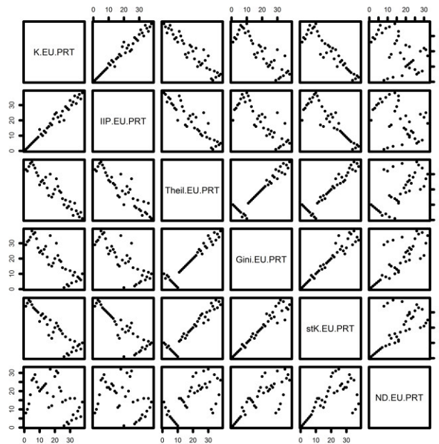
Abbildung 2 (Fortsetzung): Streudiagramme für relative Indizes
