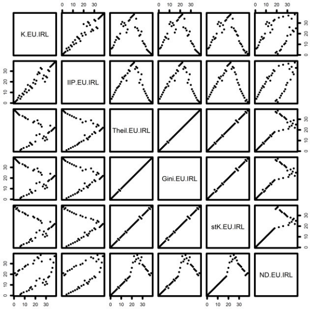
Abbildung 2: Streudiagramme für relative Indizes
