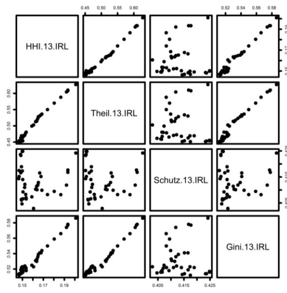
Abbildung 1: Streudiagramme für absolute Indizes
