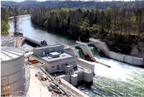
Bild 3: Wasserkraftwerk. © Pixabay https://cdn.pixabay.com/photo/2019/10/18/22/15/hydroelectric-power-station-4560237_1280.jpg 10.02.2021
