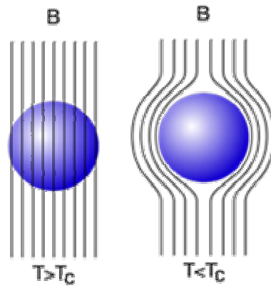
Fig. 2: Meissner-Ochsenfeld-Effect http://commons.wikimedia.org/wiki/Image:EfektMeisnera.svg
