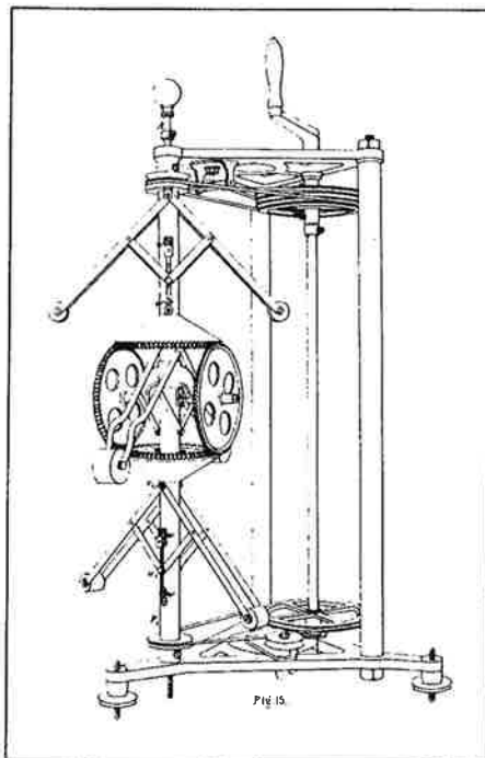
Bizykel-Modell: Mechanisches Modell zur Illustration der Wirkung zweier Stromkreise aufeinander.
