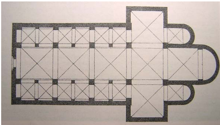
Bild 3: Grundriss einer romanischer Basilika, Quelle: http://mujweb.cz/architektura
