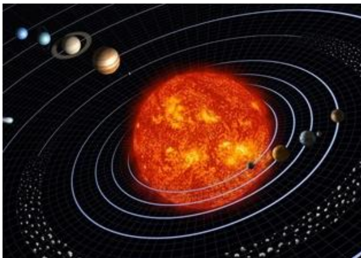
Bild 11: Sonnensystem. © Pixabay.
