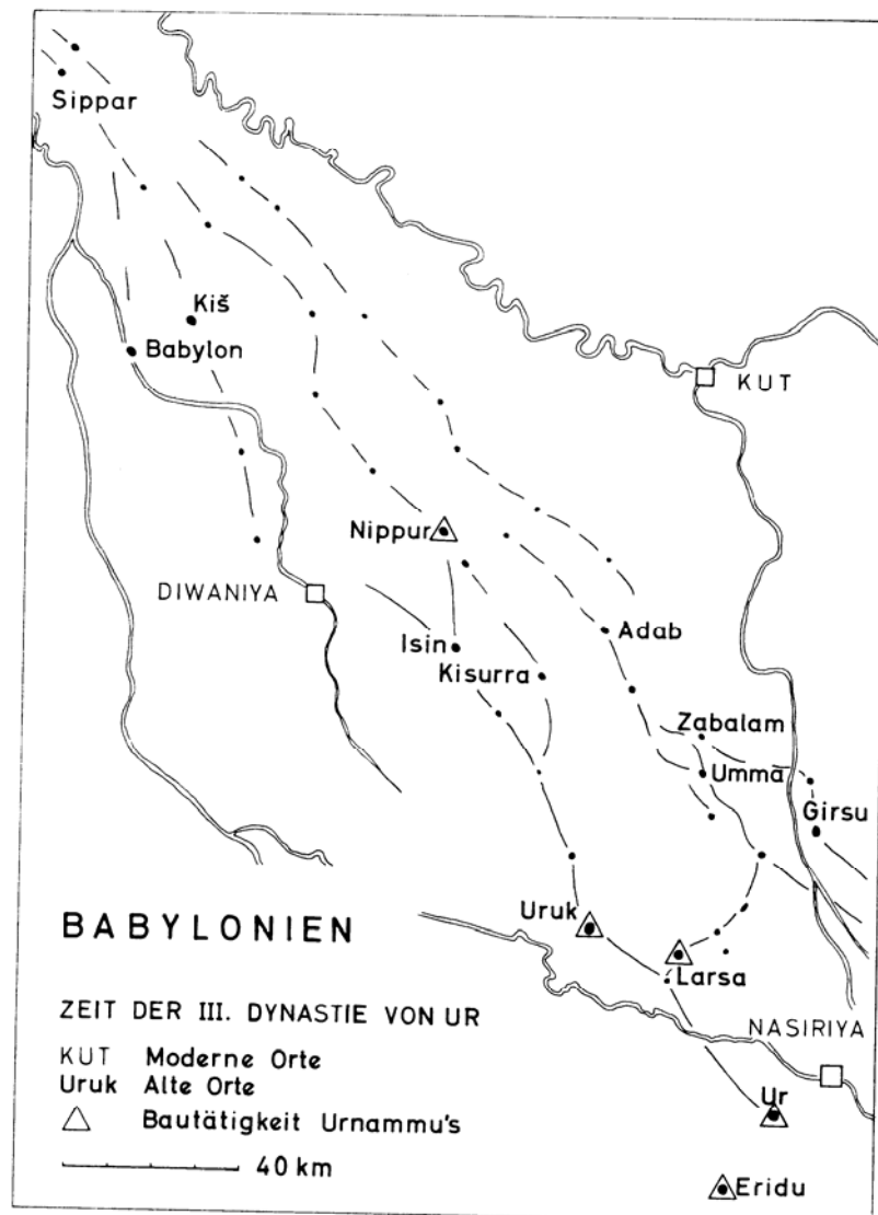
Abb. 36: Babylonien zur Zeit der III. Dynastie von UR mit Angabe der bedeutenderen Orte und Wasserläufe.
