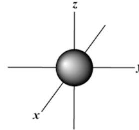
Abbildung 2.3: Abb. des kugelförmigen s-Orbitals
