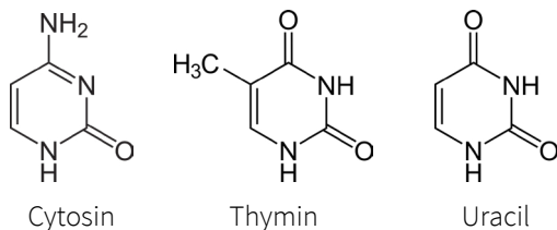
Abbildung 8.11: Die Basen sind Purin und Pyrimidin-Derivate mit unterschiedlichen Ring-substituenten
